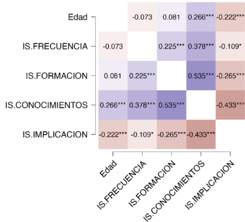
Figura 1. R de Pearson. Mapa de calor
