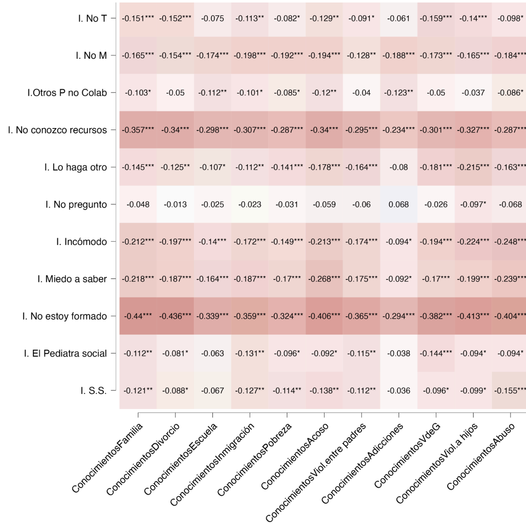
Figura 4. Mapa de color de las correlaciones entre conocimientos e implicación
