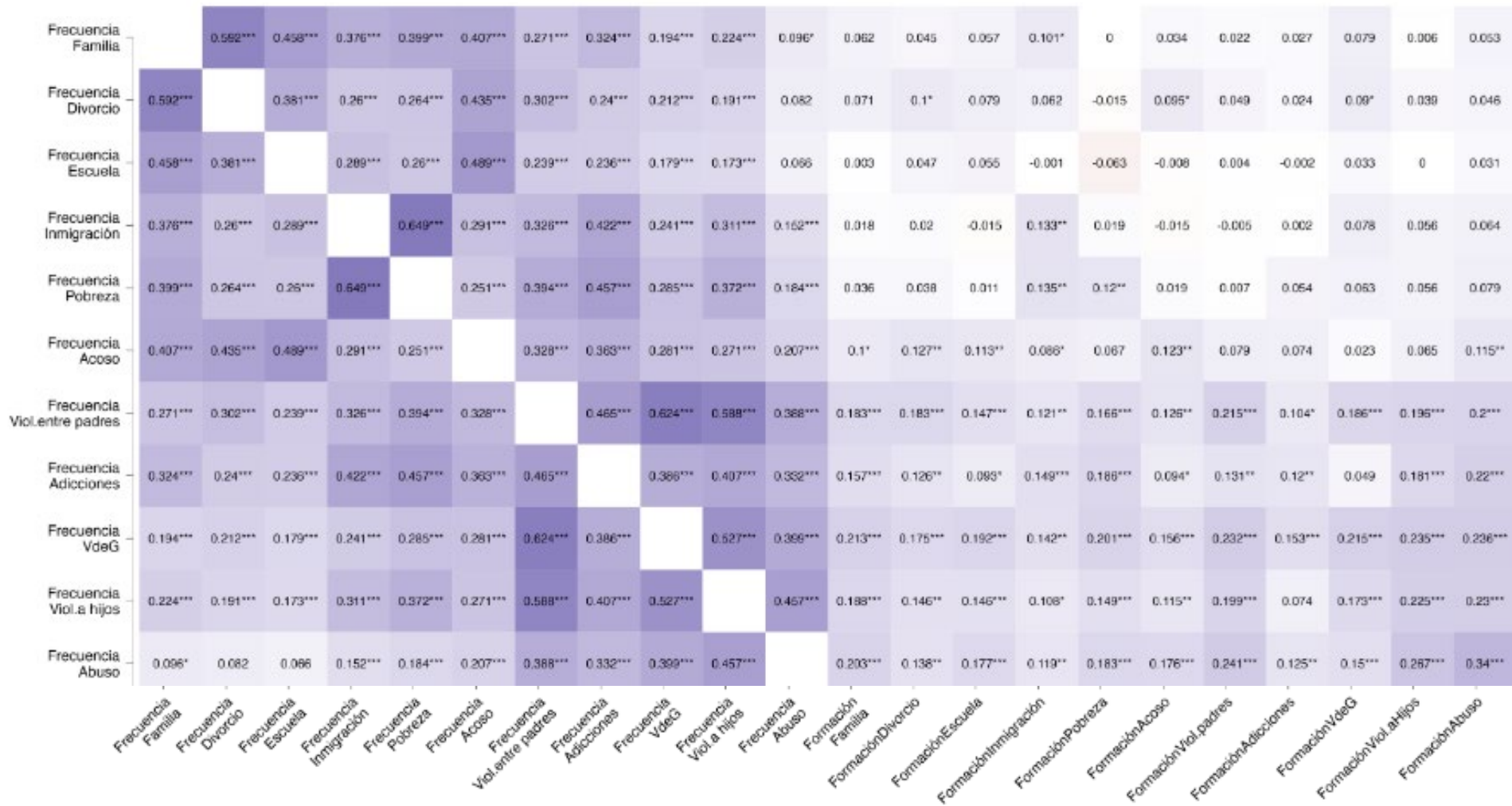
Figura 5. Tau B de Kendall. Mapa de color
